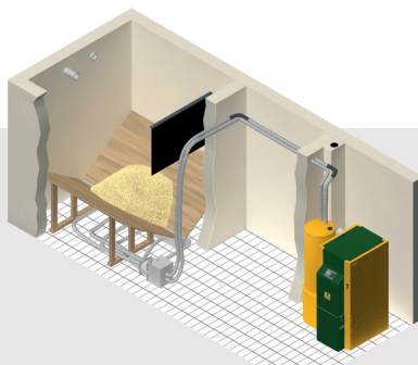
KWB UITNAMESONDES OF 1-PUNTS UITNAMESONDE MET ZUIGTRANSPORT
