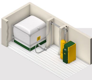
KWB-PELLETBIGBAG MET ZUIGTRANSPORT
