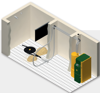
KWB PELLETROERWERK PLUS MET ZUIGTRANSPORT
