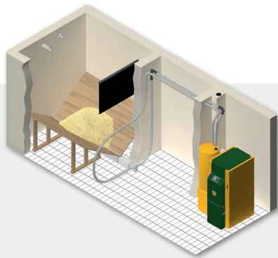
AANVOERSCHROEF MET ZUIGTRANSPORT
