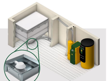
KWB-PELLETBOX MET ZUIGTRANSPORT
